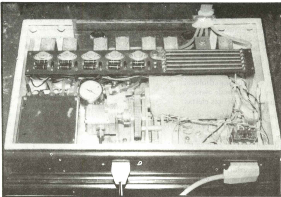
Conjunto de mecanismos instalados en la prolongación de la peana de Jesús Nazareno, para activar los movimientos del brazo.
