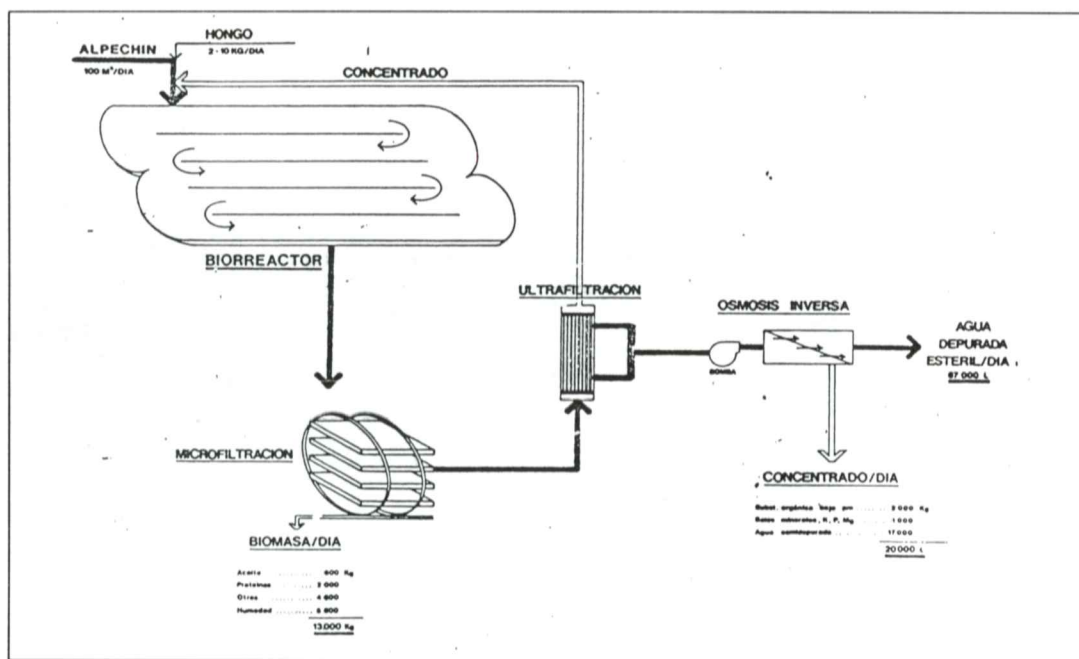
FIGURA 2. ESQUEMA PROCESO DEPURACION INTEGRAL ALPECHIN Y BALANCE DE MATERIAS
