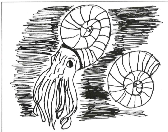
En este dibujo, realizado por Francisco Javier Sánchez Chica, se puede ver el Ammonites en su medio natural y el fósil de Ammonites.
