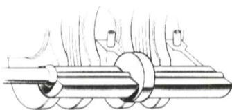
Árboles Contrarrotantes del Motor.
