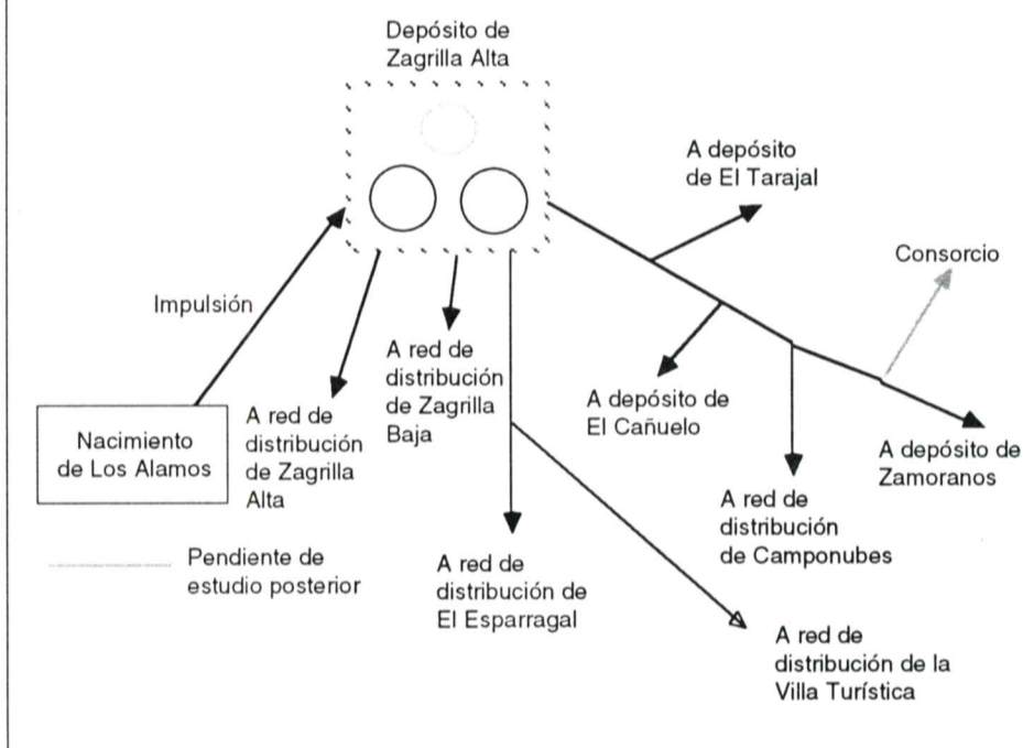
Esquema 3A. Red de abastecimiento futura de agua potable a las aldeas.
