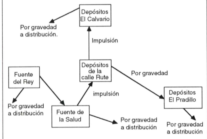
Esquema 1. Red de abastecimiento actual de agua potable de Priego.
