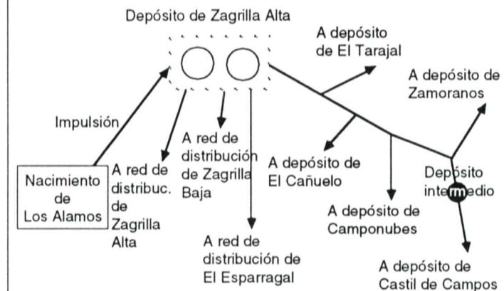
Esquema 3. Red de abastecimiento actual de agua potable a las aldeas.
