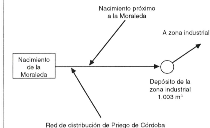
Esquema 2. Red de abastecimiento futura de agua industrial de Priego.
