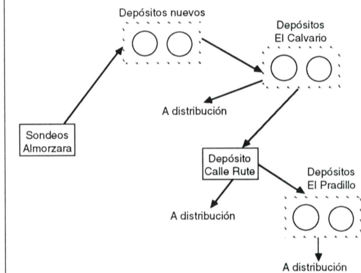
Esquema 1A. Red de abastecimiento futura de agua potable de Priego.
