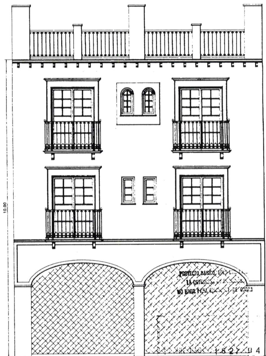
ALZADO A LA CALLE SOLANA, 6
