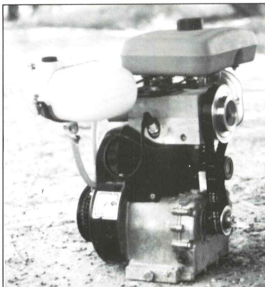
Motor de 4 tiempos con "culata sin válvulas".
