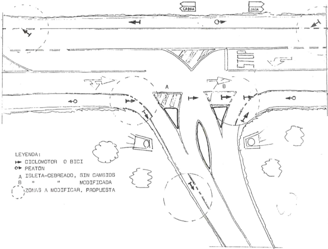
Croquis 1. Propuesta de adaptación de marcas viales y de borde: ciclomotores y bicicletas.
