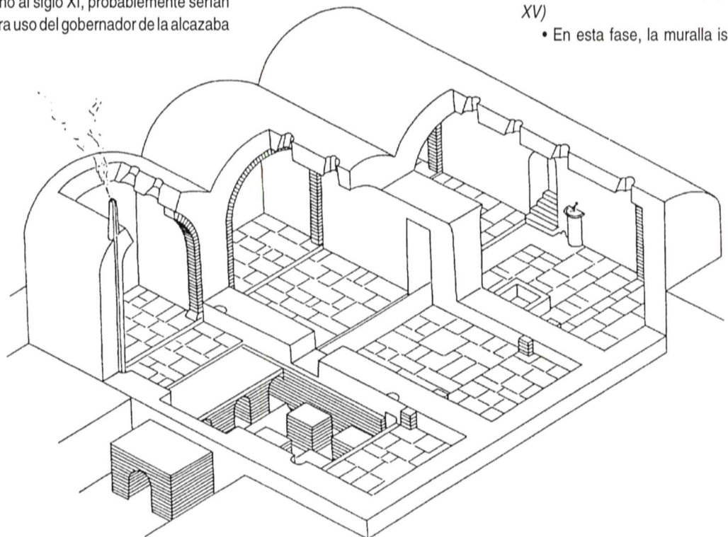
Reconstrucción de unos baños árabes andalusíes, donde se aprecia perfectamente la disposición original de la sala de baños calientes y su sistema de calefacción mediante pilares bajo el pavimento de la estancia, tal como se ha documentado en el castillo de Priego.
