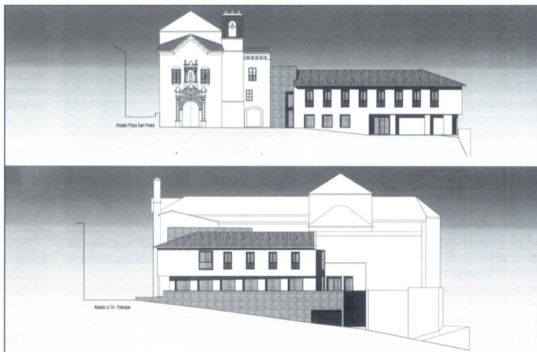
Alzado frontal y lateral del nuevo edificio
