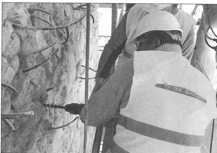
Un momento del cosido de la estructura medieval, el proceso de obra más complejo y técnico
