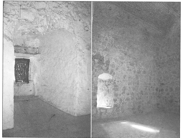
Ejemplo de recuperación de ventana aspillerada medieval, antes y después
