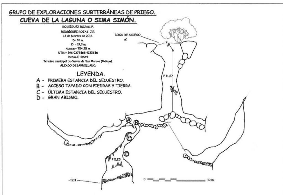
Alzado topográfico de la cueva
